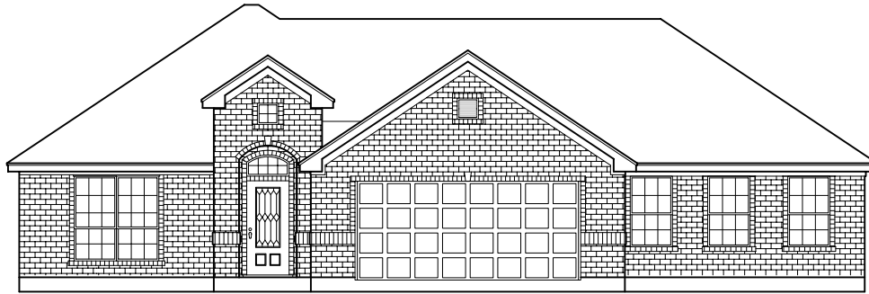
ELEVATION A
